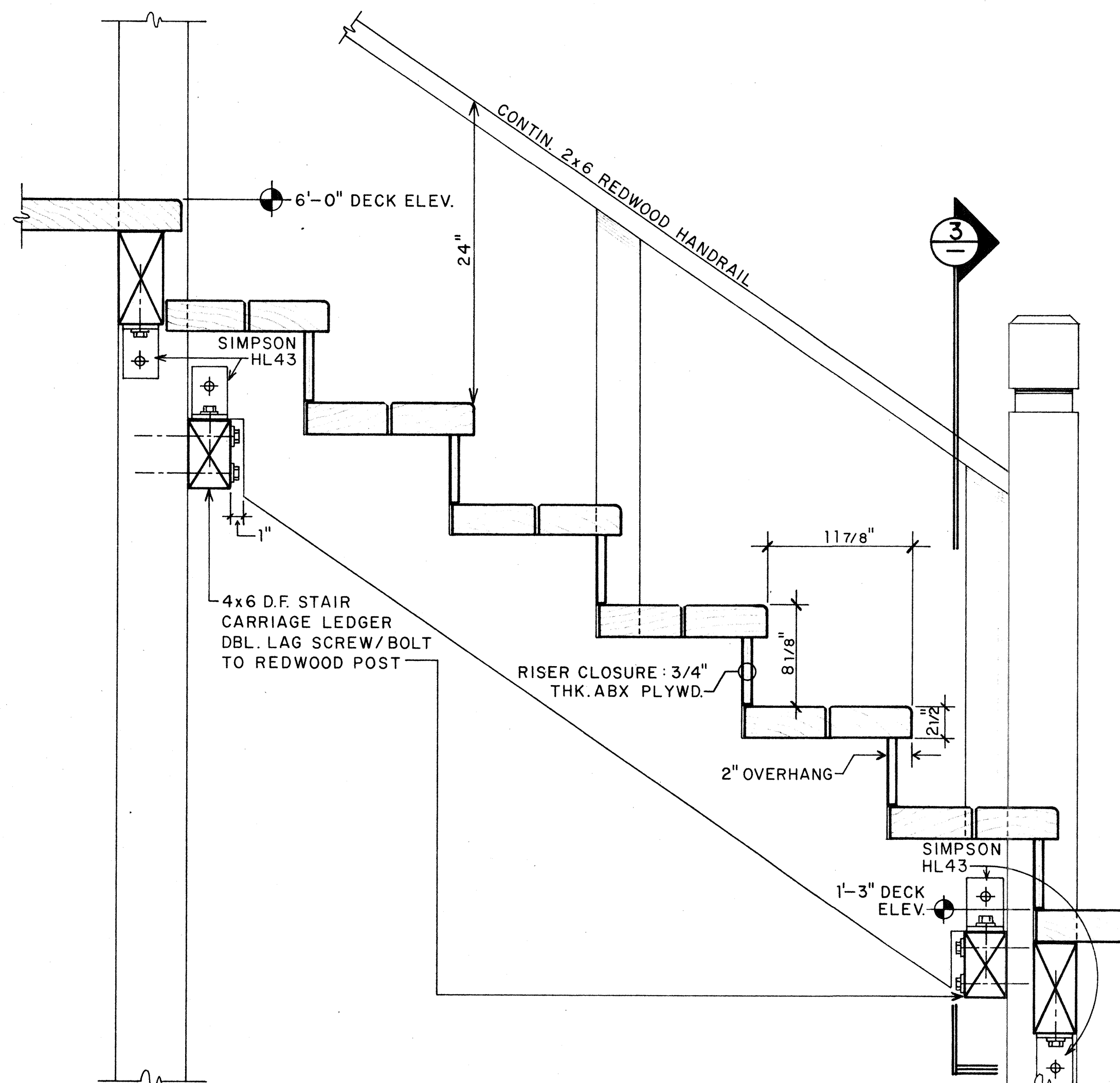
LONGITUDINAL STAIR SECTION
